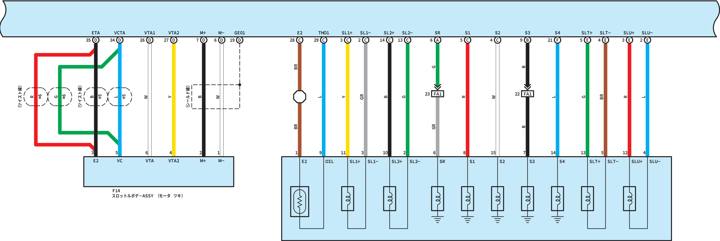
F44 ECT ソレノイド
